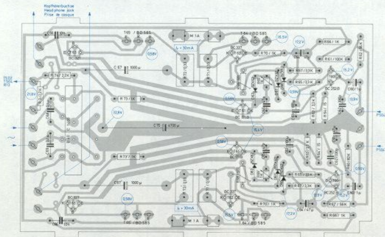
Fig. 9 Endverstärker 227 587 (Leiterseite)
